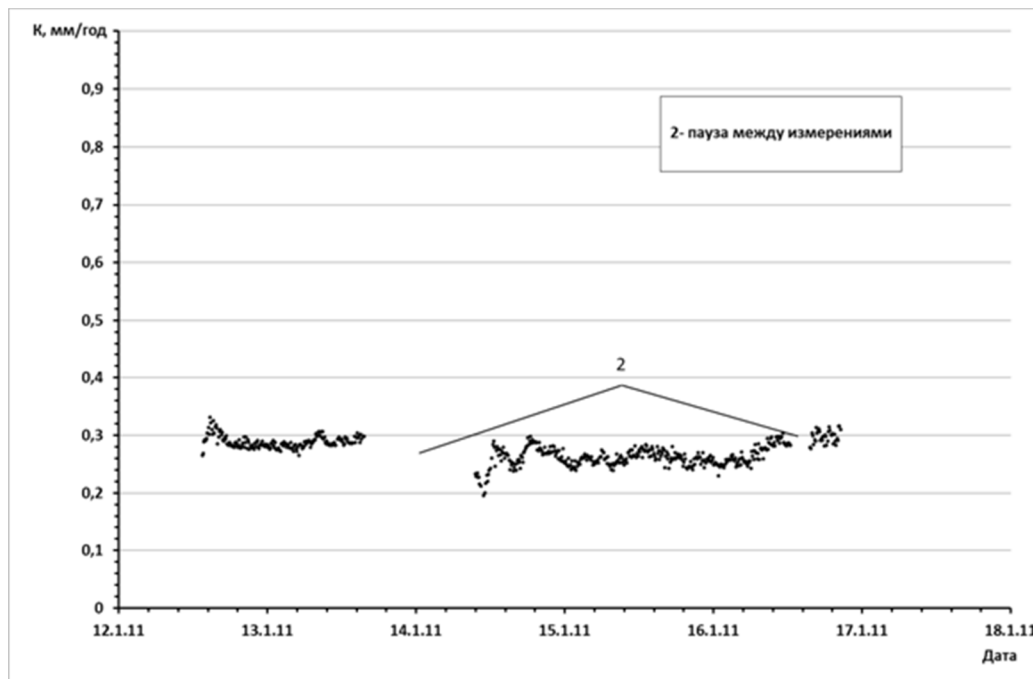
Рис.6 Скорость коррозии проволоки из Ст3 при испытаниях в 3%-ном растворе NaCl при анодном растворении при 25°C. Масштаб скорости коррозии 0 – 1 мм/год
