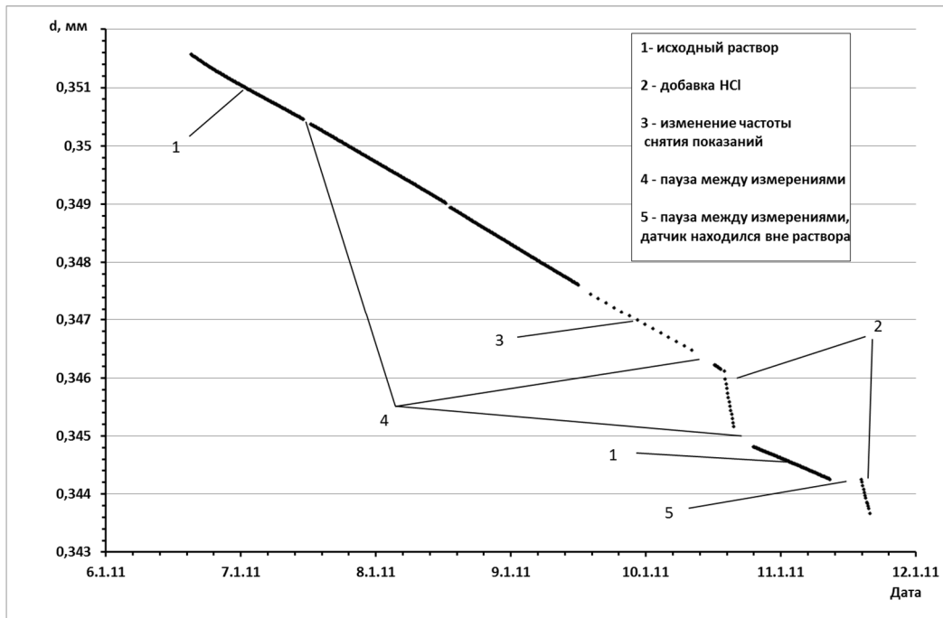
Рис.2 Изменение диаметра проволоки из Ст3 при испытаниях в 3%-ном растворе NaCl с добавками HCl при 25°C
