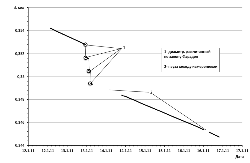
Рис.4 Изменение диаметра проволоки из Ст3 при испытаниях в 3%-ном растворе NaCl при анодном растворении при 25°C
