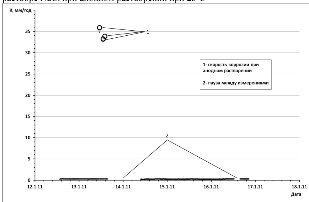
Рис.5 Скорость коррозии проволоки из Ст3 при испытаниях в 3%-ном растворе NaCl, в т.ч. при анодном растворении при 25°C. Масштаб скорости коррозии 0-40 мм/год
