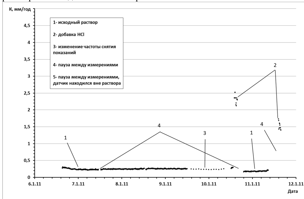
Рис.3 Скорость коррозии проволоки из Ст3 при испытаниях в 3%-ном растворе NaCl с добавками HCl при 25°C
