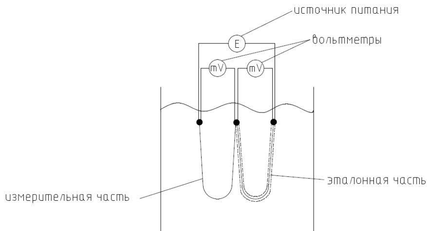
Рис.1 Функциональная схема измерения скорости коррозии методом электрического сопротивления
